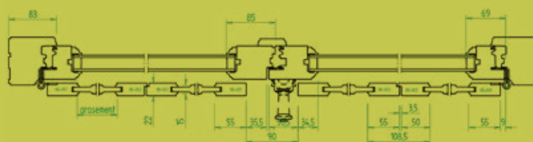
COUPE HORIZONTALE
